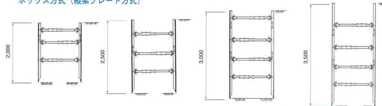
ボックス方式（縦梁プレート方式）
