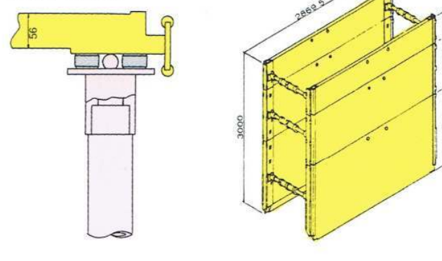
ボックス方式
