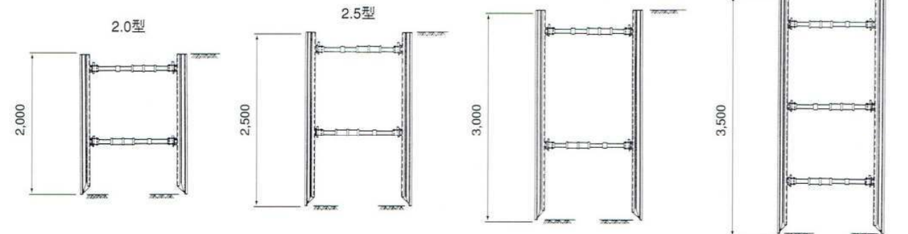
ボックス方式（縦梁プレート方式）
