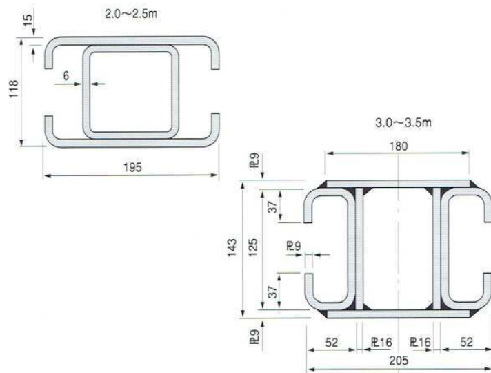
レール断面
